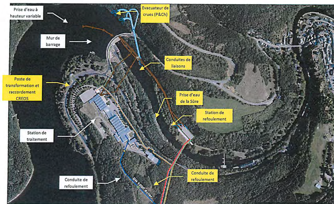
Annexe 1 : Équipements existants (blanc) et des nouveaux équipements (jaune) à Esch-sur-Sûre
