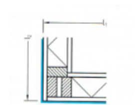
Figure 27: plus grande longueur développée l = l_1 + l_2
