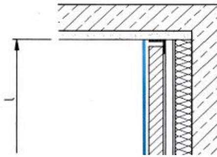
Figure 61: Coupe horizontale sur façade ; angle rentrant - céramique / enduit
