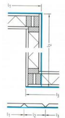
Figure 26: plus grande longueur développée l = l_1 + l_2 + l_3
