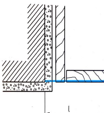
Figure 101 : Surfaces limitées par un élément de construction
