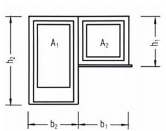
Figure 72: Réservations de même nature
