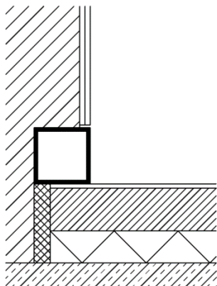
Figure 103 : plinthe à calculer séparément
