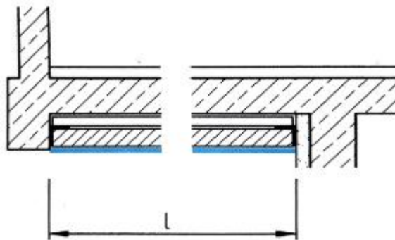
Figure 63: Sous-face de balcon ; coupe verticale céramique / enduit
