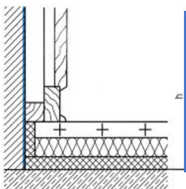
Figure 100 : Surfaces limitées par un élément de construction –
